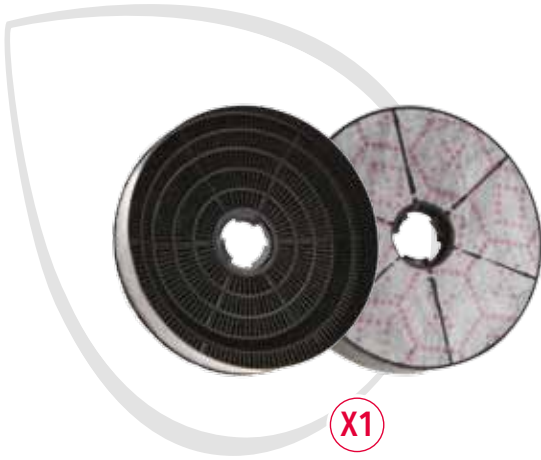
KFC6918 (CP178) 35602061 EAN 8016361972940 Ø170x35mm; 180gr - Tipo 178
