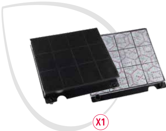
KFC6912 (CPM15) 35602055 EAN 8016361971288 225x210x30mm; 530gr - Tipo M15
