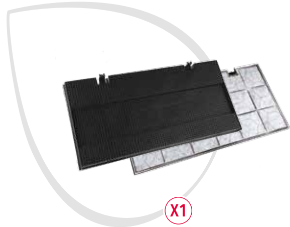
KFC6911 (CP150) 35602054 EAN 8016361971271 435x217x20mm; 1110gr - Tipo 150
