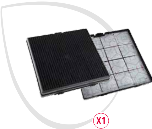
KFC6910 (CP241) 35602053 EAN 8016361971264 223x228x30mm; 510gr - Tipo 241
